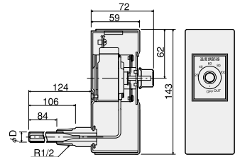
●EAC-3LT, 4LT寸法図
