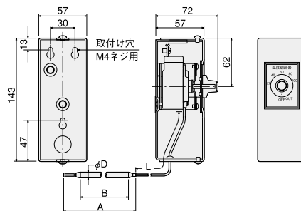
●寸法図
