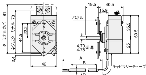
●寸法図
