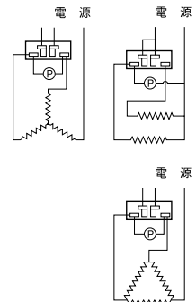
●配電図
