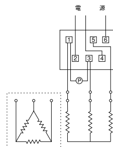
● 配電図
