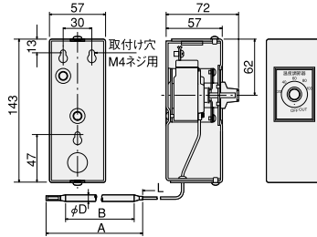
●EAC寸法図
