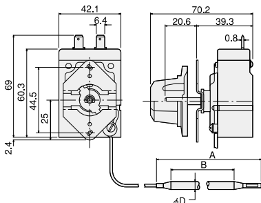
●寸法図
