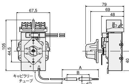
● 寸法図
