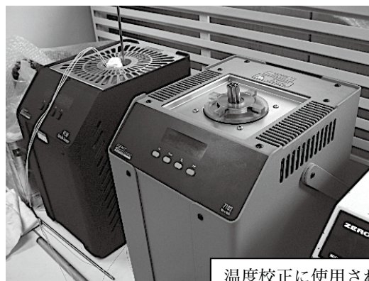
温度校正に使用されるバス (恒温器) です。
